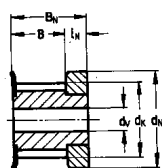
Ausführung 1
