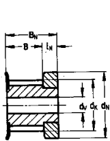
Ausführung 1
