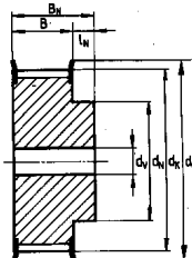
Ausführung - 2
