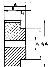
Ausführung - 0
