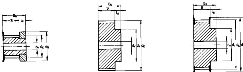
Ausführung 1
