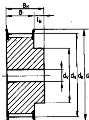
Ausführung - 2
