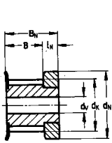
Ausführung 1
