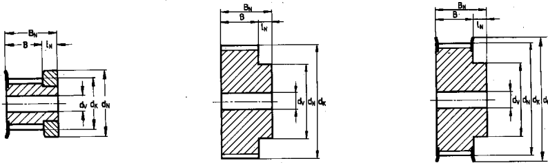
Ausführung 1
