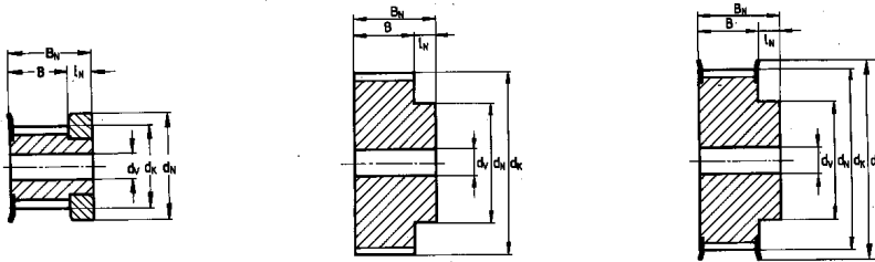
Ausführung 1
