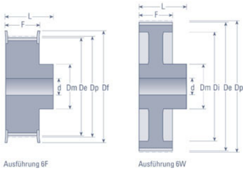
Ausführung 6F
