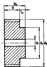
Ausführung - 0
