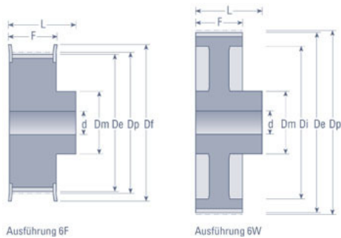
Ausführung 6F
